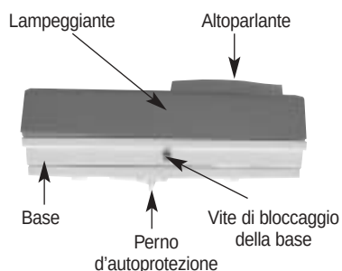
Vista dal basso della sirena
