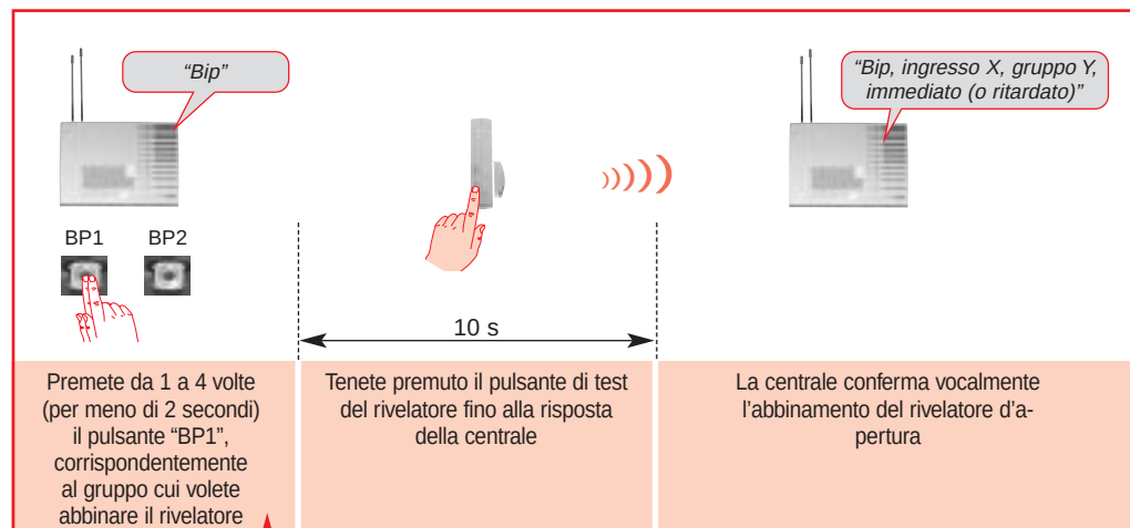
BP1 (solo per l'abbinamento dei rivelatori d'apertura)
