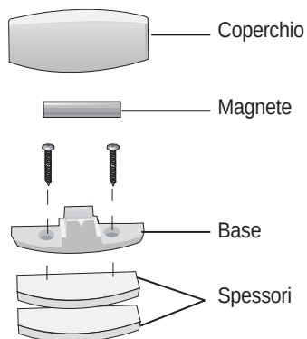
Fig. C - Montaggio del portamagnete
