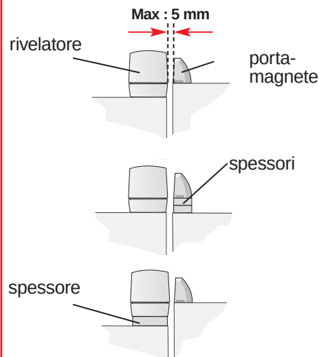
Fig. B - Regolazione dell'altezza
