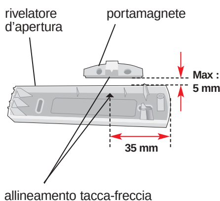
Fig. A - Allineamento
