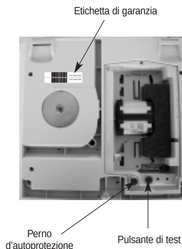
Vista interna della sirena
